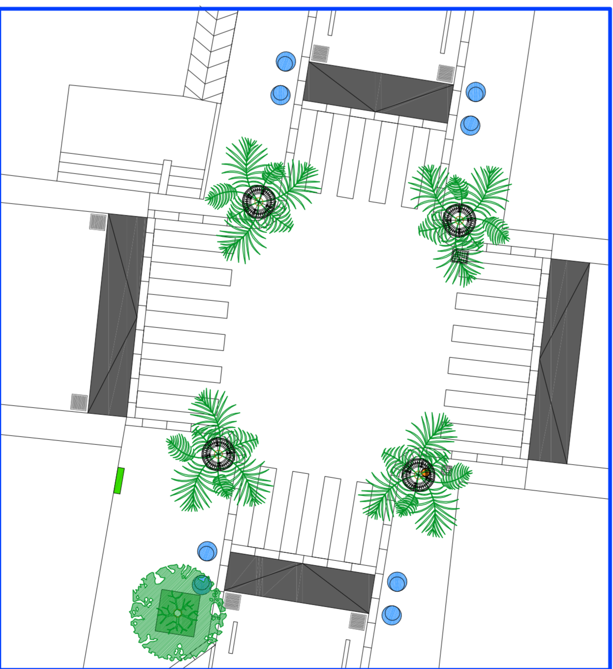
Schema di una intersezione sopraelevata
