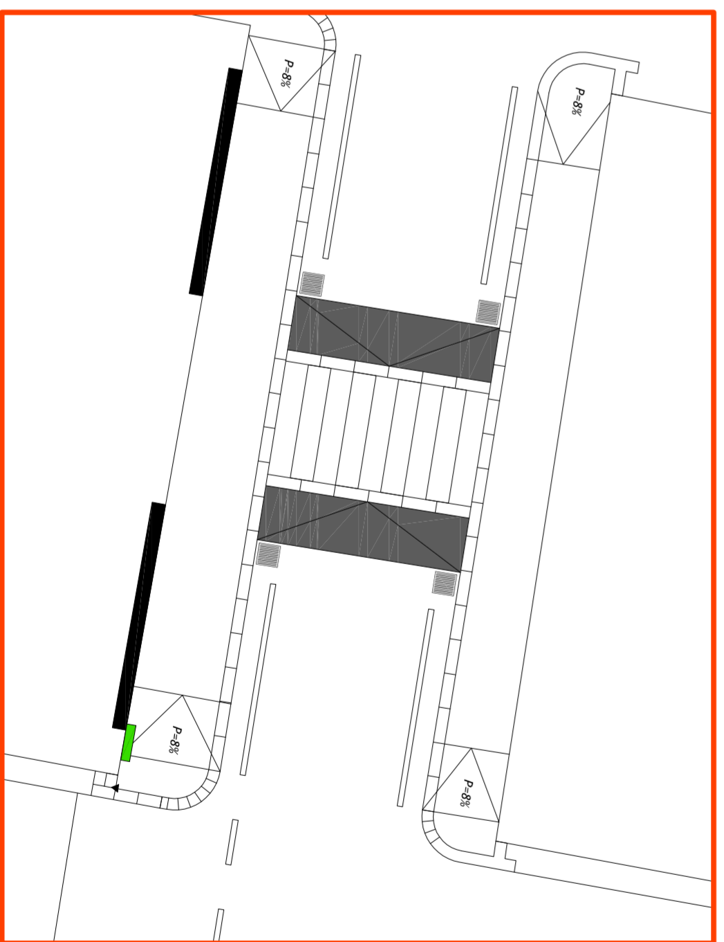
Schema di un attraversamento pedonale protetto
